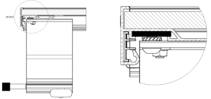
Fixation des consoles de coulissement haute
